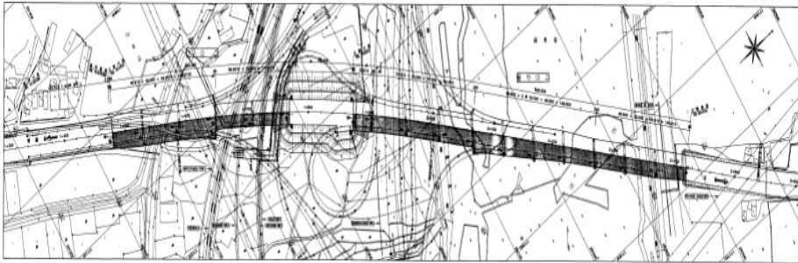
<그림 6.21>범안대교(안심방향) 평면도
